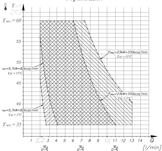
G-23-03 AQUA COMFORT turbo o výkone 23kW
