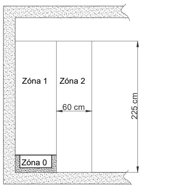
obr.3.1.1.2 Bočný pohľad - sprcha
