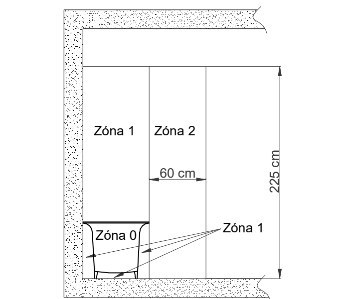
obr.3.1.1.1 Bočný pohľad - vaňa
