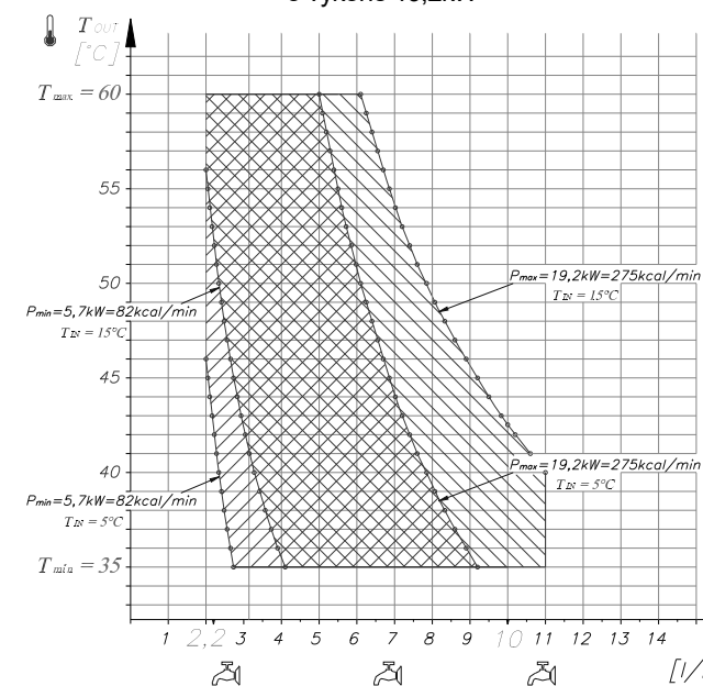
GT-19-03 AQUA COMFORT turbo o výkone 19,2kW
