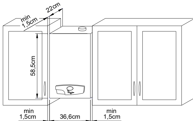
obr. 3.3.1. Požadované montážne rozmery
