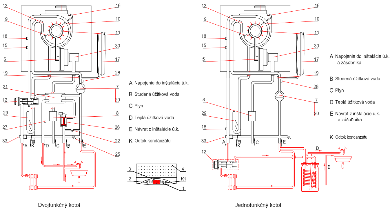
Dvojfunkčný kotel
