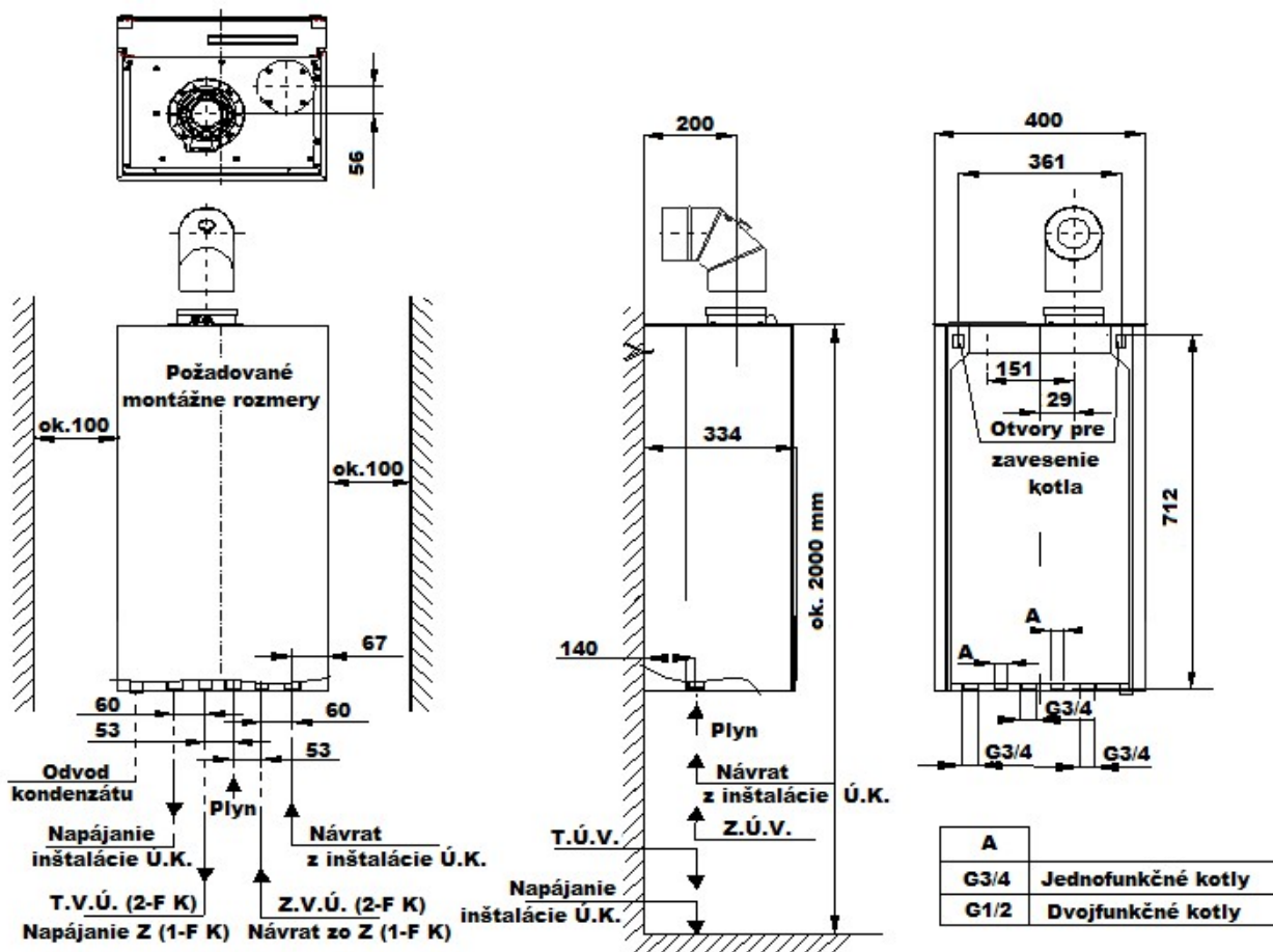
Obr. 3.3.1 Inštalačné rozmery kotlov ECOCONDENS SILVER PLUS
