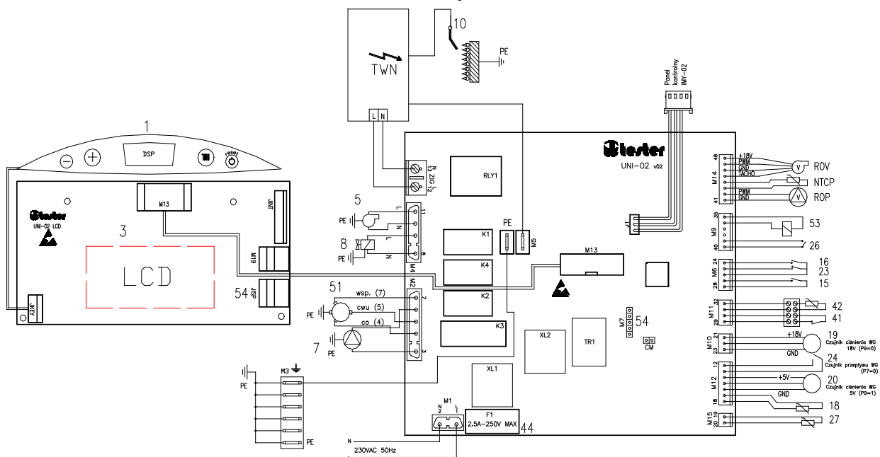
Dvojfunkčný kotol
