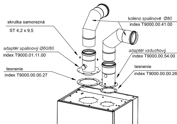
Oddelený systém (nezávislý) – názorný obrázok pre potrubia vzduchovo – spalinové kovové
