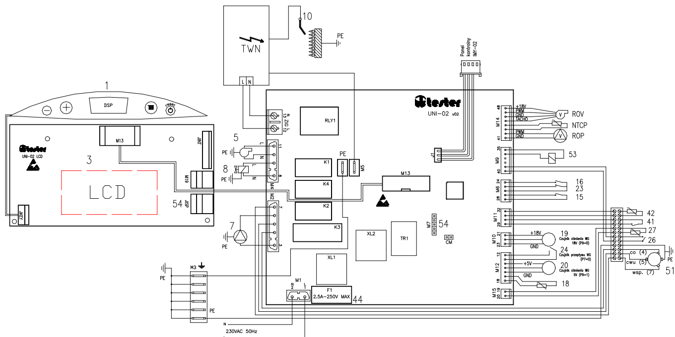
Jednofunkčný kotol
