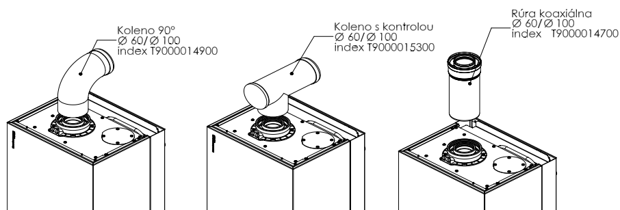
Koaxiálny systém – názorné obrázky pre potrubia vzduchovo – spalinové plastové
